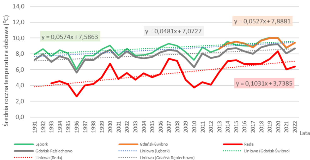
Rys.1. Wieloletnia zmienność średniej rocznej dobowej temperatury powietrza, Reda, Łębork, Gdańsk-Świbno, Gdańsk-Rębiechowo
