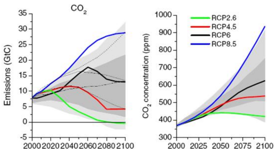
Rys.40. Różnice projekcji emisji CO 2 (lewy panel) i prognozowanych stężeń CO 2 (prawy panel) pomiędzy scenariuszami RCP. Obszar zacieniowany odpowiada 98. i 90. percentylowi (jasny i ciemny szary) – dane z literatury
