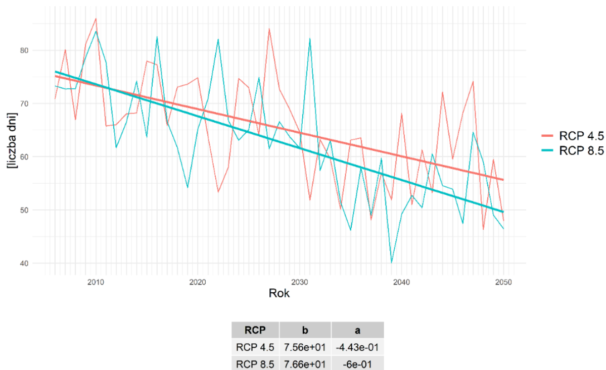
Rys.59. Liczba dni przymrozkowych ( T_{\min} < 0^{\circ}\text{C} ), uśredniona dla obszaru Miasta Reda
